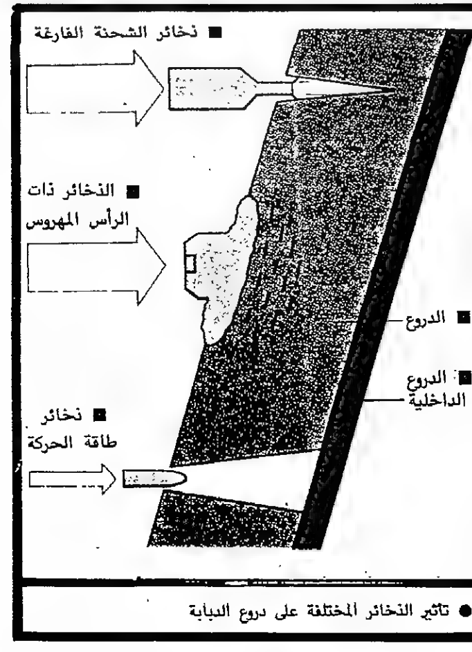
● تأثير الذخائر المختلفة على دروع الدبابية
